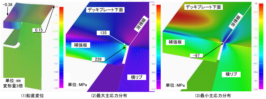
図-5 鉛直変位および最大・最小主応力, D(8, 75, infinity, 60, 9)モデル
